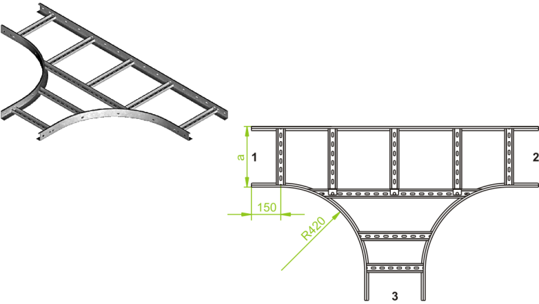
Przy różnych szerokościach drabin należy podać wymiary 1,2,3.
